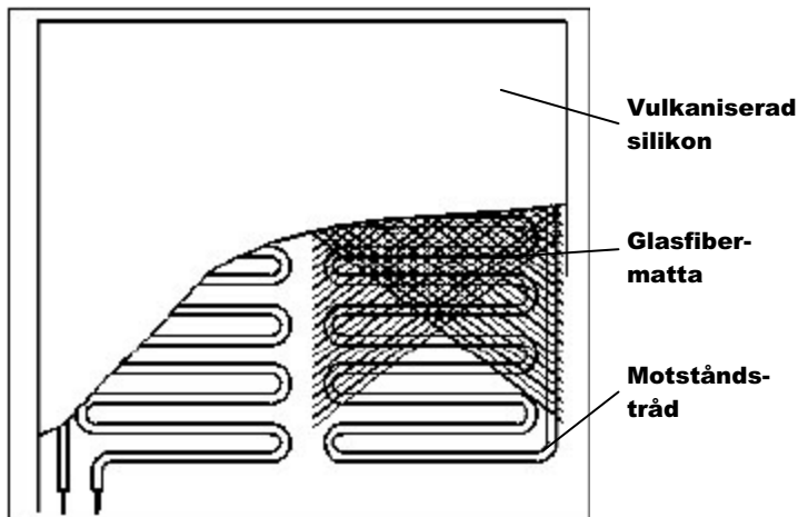
Uppbyggnad av en silikonmatta.
