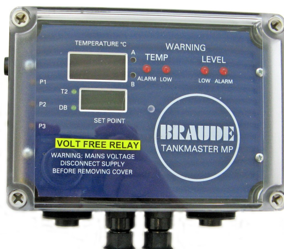
Kombinerad nivåvakt och temperaturstyrning
